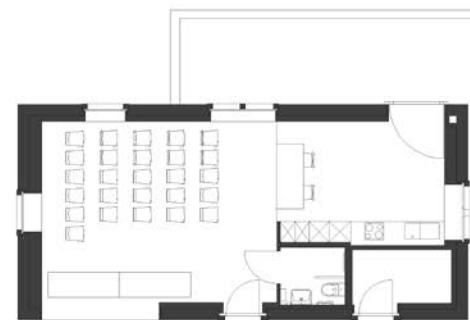
Reihenbestuhlung 26 Pers.
